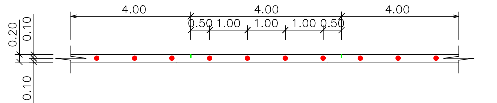
VÝREZ Z PŮDORYSU CB DOSKY – OBRATISKO A ODSAVNÁ PLOCHA PRE BUS KÓTOVANÉ V m
