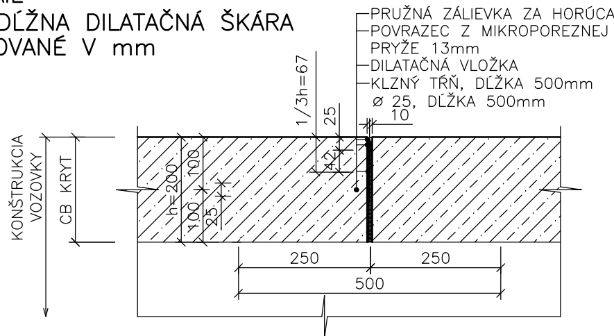
DETAIL "A" PRIEČNA ŠKÁRA KÓTOVANÉ V mm
