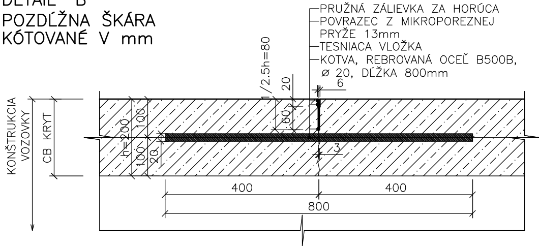
DETAIL PRIEČNA DILATAČNÁ ŠKÁRA KÓTOVANÉ V mm
