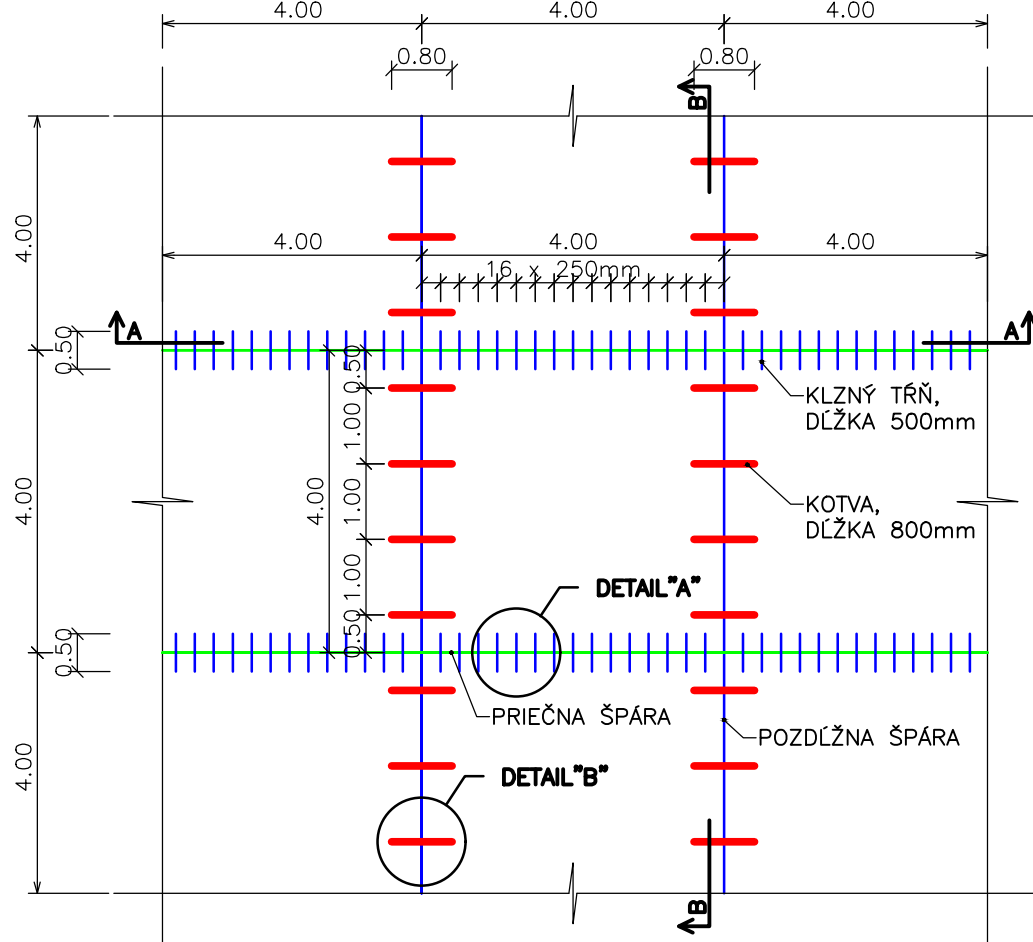
VÝREZ Z PŮDORYSU CB DOSKY – OBRATISKO A ODSAVNÁ PLOCHA PRE BUS KÓTOVANÉ V m
