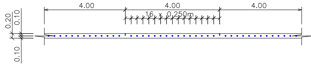
REZ CB DOSKOU B–B KÓTOVANÉ V m
