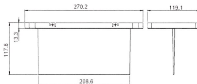
SafeLite - oboustranný panel s bezpečnostní značkou
