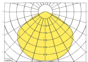
Křivka svítivosti
