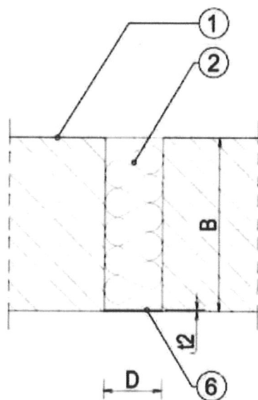
Obr. B3. Tesnenie lineárneho spoja v pevnej stene s použitím minerálnej vlny a Flame Cabel A Paste.
