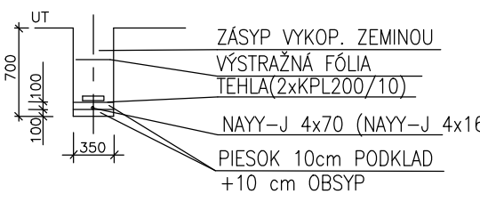
ULOŽENIE KÁBLA VO VOLNOM TERÉNE M 1:50
