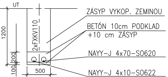
ULOŽENIE KÁBLA POD KOMUNIKÁCIU A-A M 1:50
