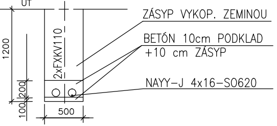
ULOŽENIE KÁBLA POD KOMUNIKÁCIU B-B M 1:50
