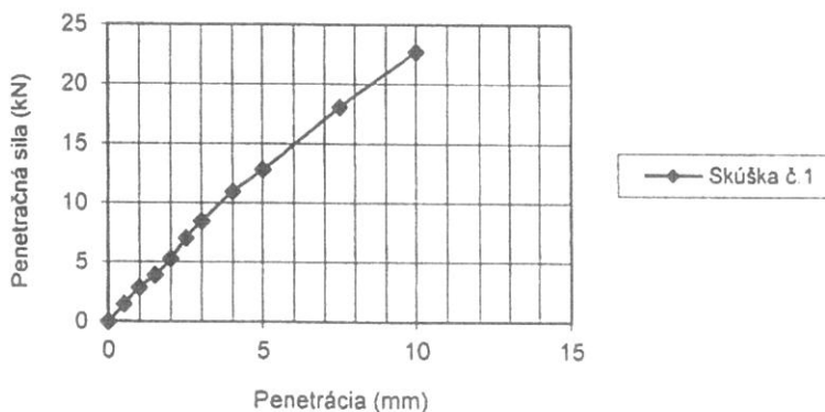
Závislosť penetrácie od penetračnej sily
