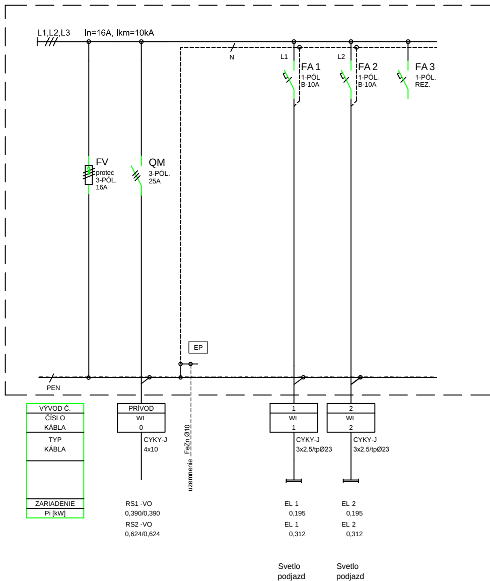
JEDNOPÓLOVÁ SCHÉMA ROZVODNICE RS1(2)-PODJAZD
