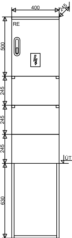
ROZVÁDZAČ RS1(RS2) ROZMEROVÝ NÁČRT M 1:50
